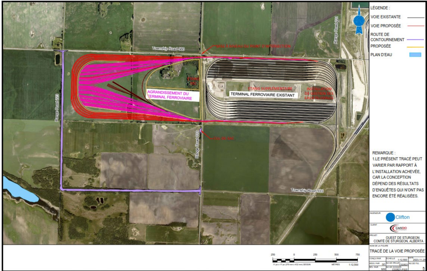
Figure 5 – Disposition des voies proposée
