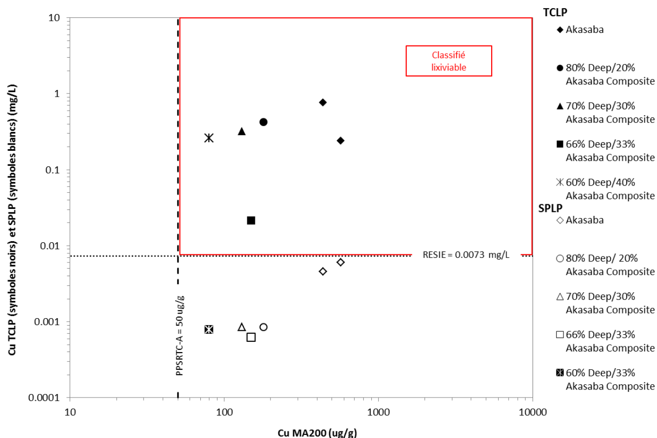
Figure 9: La concentration en cuivre (mg/L) dans les lixiviats TCLP en fonction du contenu en cuivre extractible (ug/g) des échantillons de résidus.
