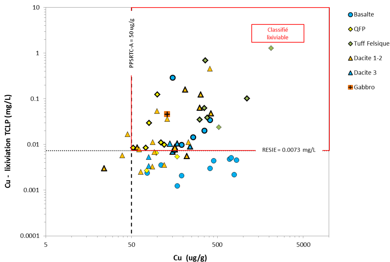
Figure 5 : La concentration en cuivre (mg/L) dans les lixiviats TCLP en fonction du contenu en cuivre extractible (ug/g) des échantillons de roches stériles. Les symboles des échantillons de roches stériles utilisés pour construire les colonnes de lixiviation (basalte, QFP et tuf) et la cellule d'humidité (gabbro) ont un contour noir gras.
