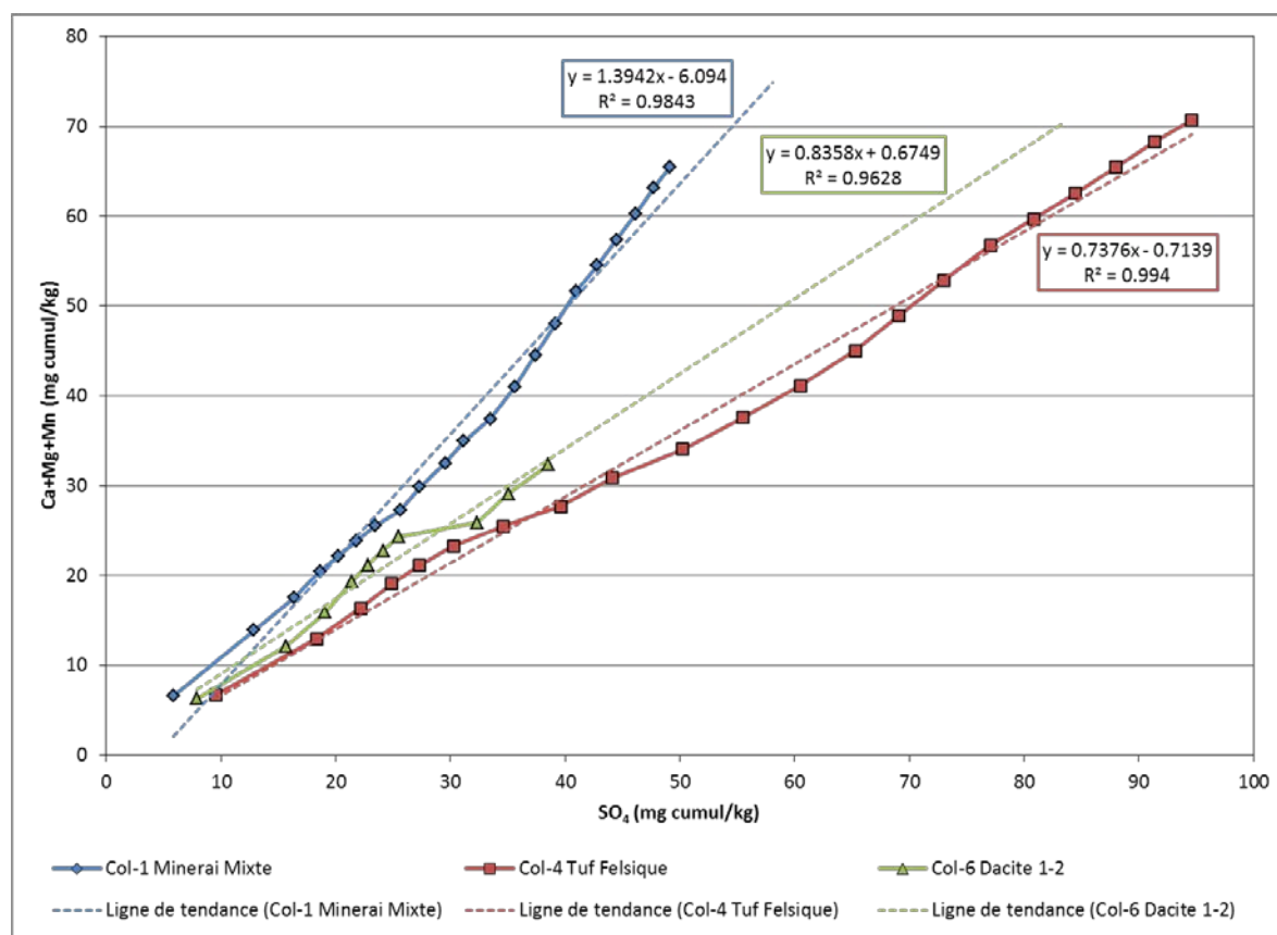
Figure 10: Courbes d'oxido-neutralisation des échantillons de stériles PGA soumis à l'essai cinétique en colonne.
