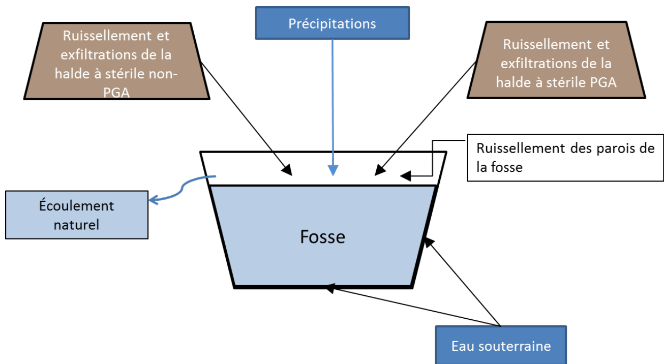
Figure 12: Bilan d'eau de la fosse en période postfermeture.
