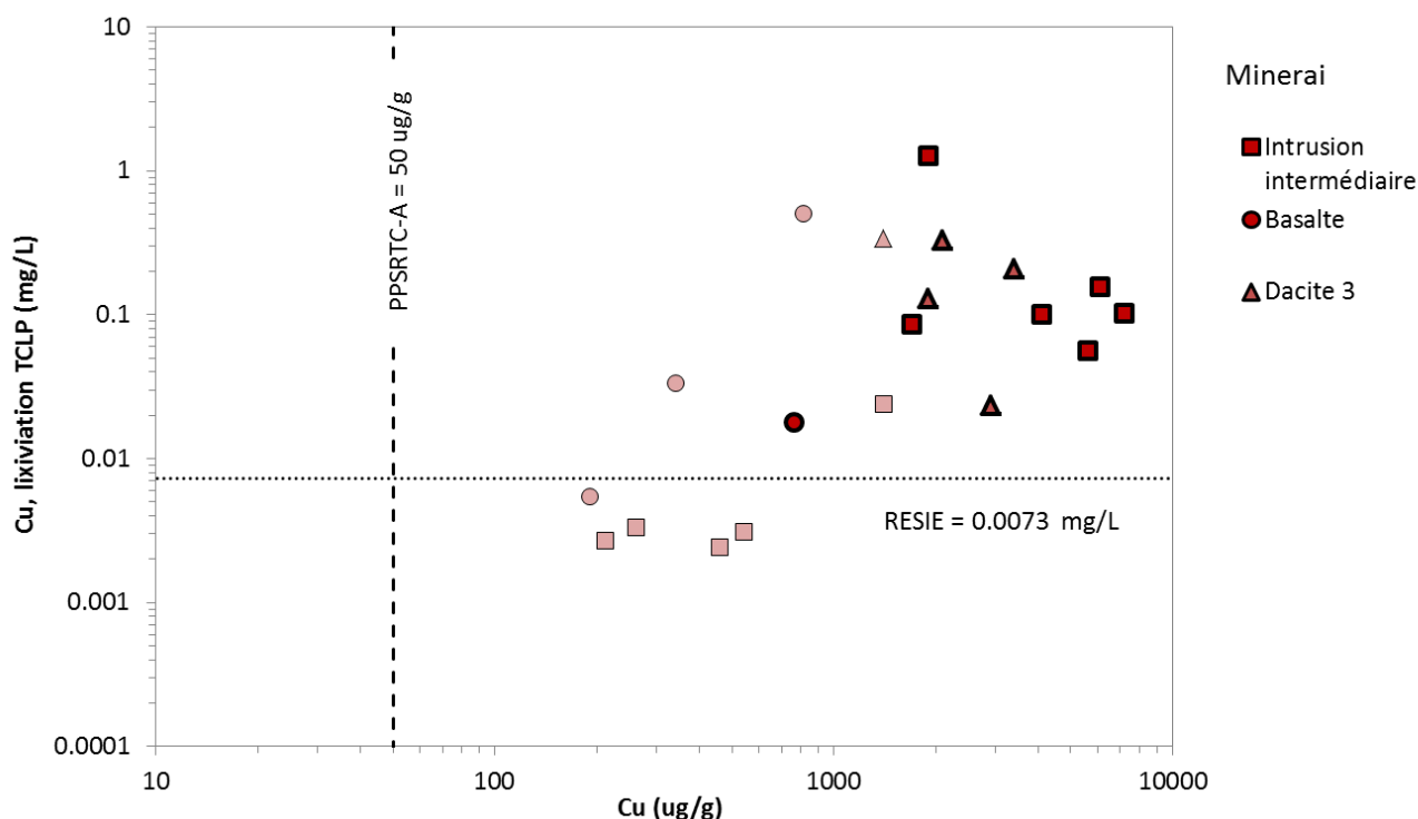
Figure 6 : La concentration en cuivre (mg/L) dans les lixiviats TCLP en fonction du contenu en cuivre extractible (ug/g) des échantillons de minéral. Les symboles des échantillons de minéral pour construire la colonne de lixiviation de minéral mixte ont un contour noir gras.
