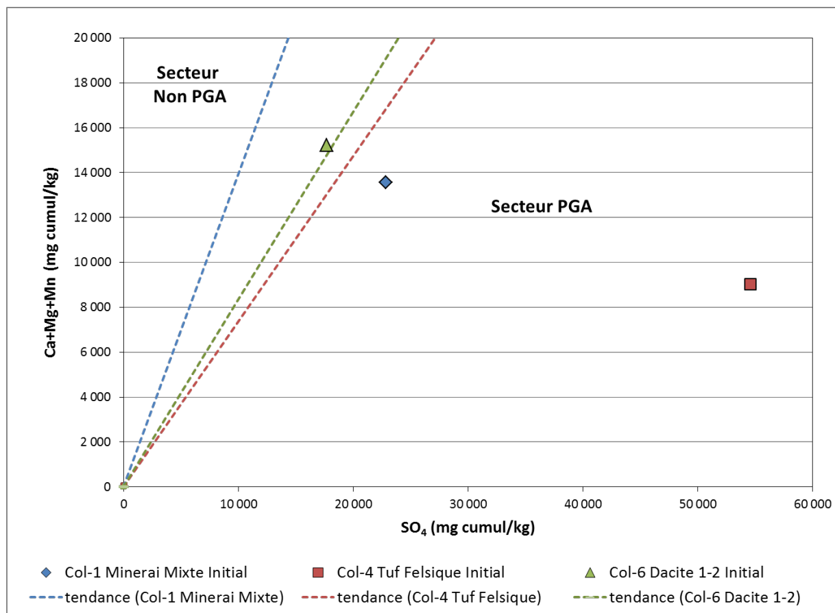
Figure 11: La propension à l'éventuelle acidification des stériles PGA selon la comparaison des taux de lixiviation des composés indicateurs d'oxydation et de neutralisation et la composition initiale de chaque échantillon.
