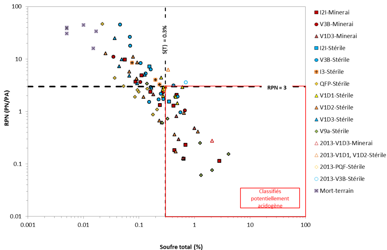
Figure 7: Le RPN en fonction du soufre total (%) pour les échantillons de minéral et de stérile
