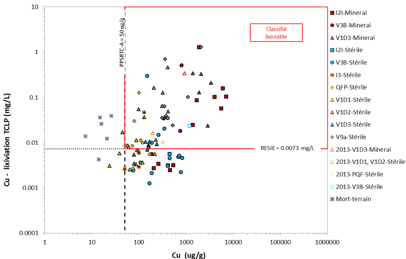
Figure 8: La concentration en cuivre (mg/L) dans les lixiviats TCLP en fonction du contenu en cuivre extractible (ug/g) des échantillons de minerai et de stériles.
