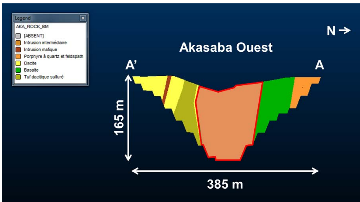
Figure 3: Coupe géologie A-A¹ de la fosse prévue (modifié de AEM comm. pers. 2014-2015).
