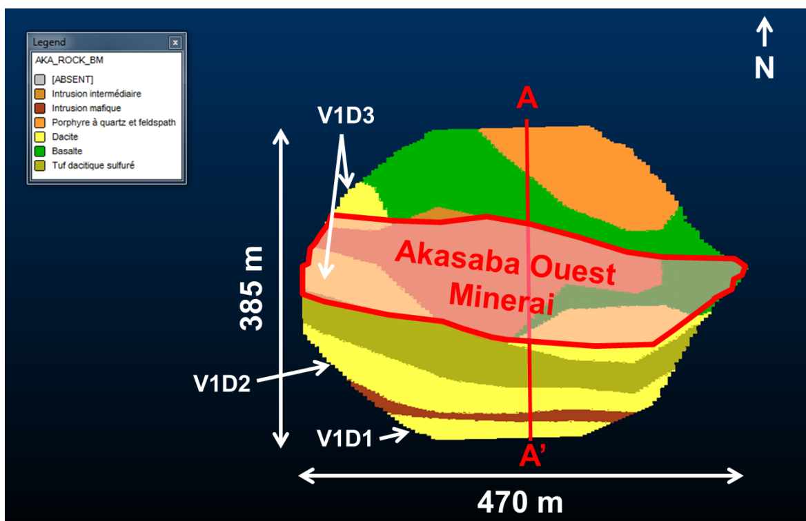
Figure 2: Schéma et géologie de la fosse prévue (modifié de AEM comm. pers. 2014-2015).
