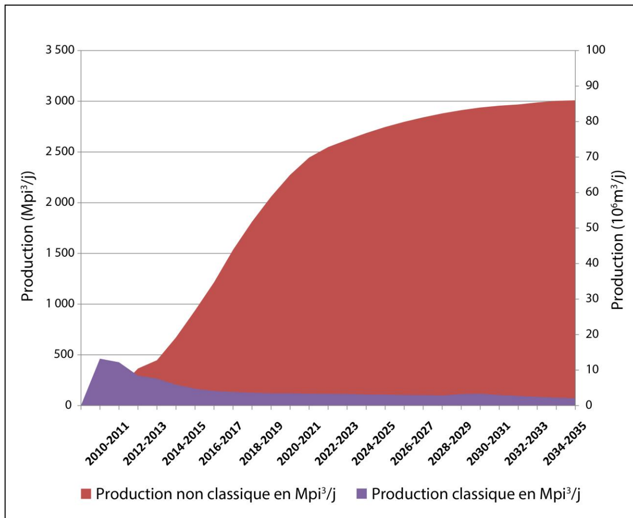
Figure 4-2: Production de NGTL prévue pour la région de North Montney
