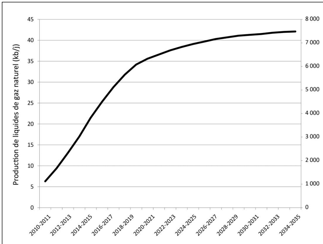
Figure 4-3 : Production prévue de liquides de gaz naturel dans la région de North Montney
