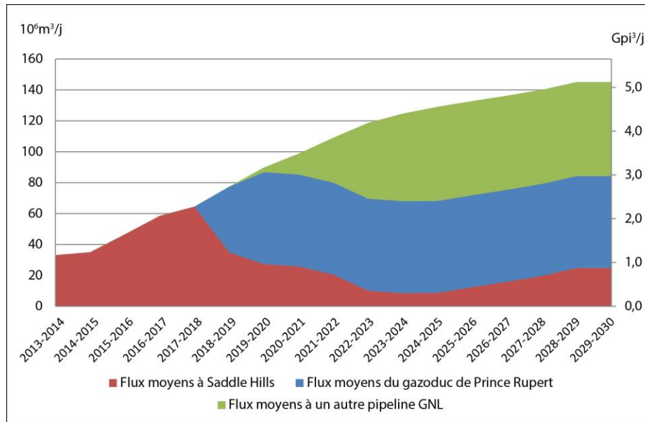
Figure 4-6 : Moyennes prévues de flux gaziers de livraison dans le territoire désigné
