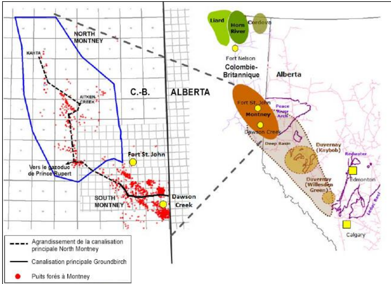
Figure 4-1 : Bassin d'exploitation North Montney de NGTL
