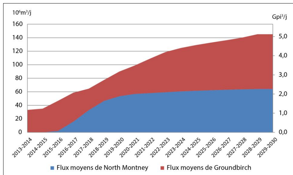
Figure 4-5 : Moyennes prévues de flux gaziers de réception dans le territoire désigné
